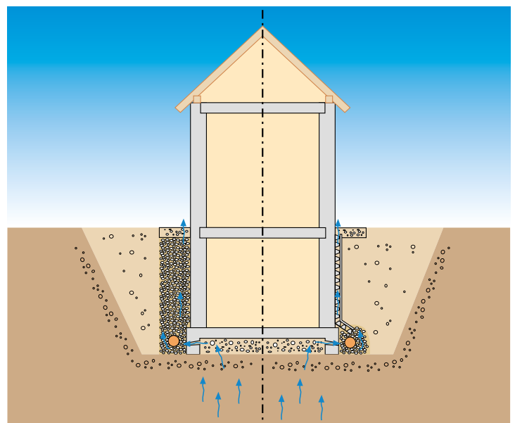
Traditionelle Gasflächendrängung und Lösung mit DELTA®-GEO-DRAIN QUATTRO/DELTA®-TERRAXX.
