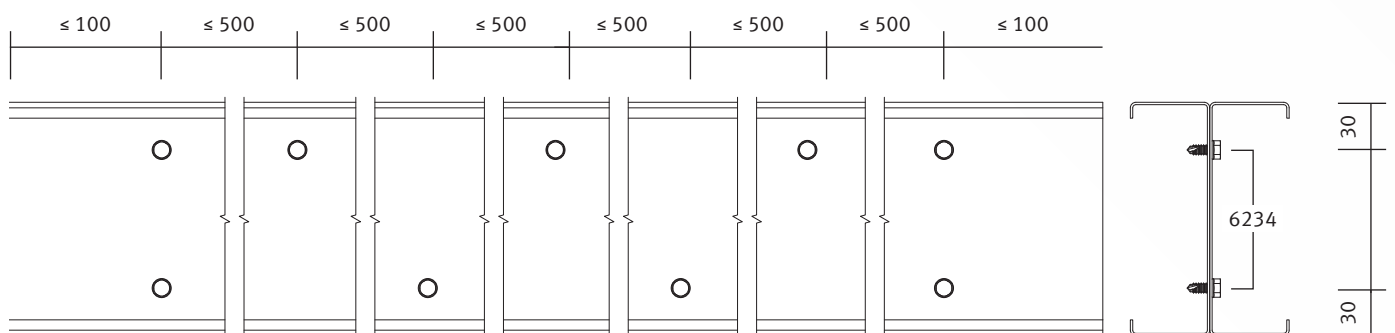
Verschraubung der Weitspannträger
