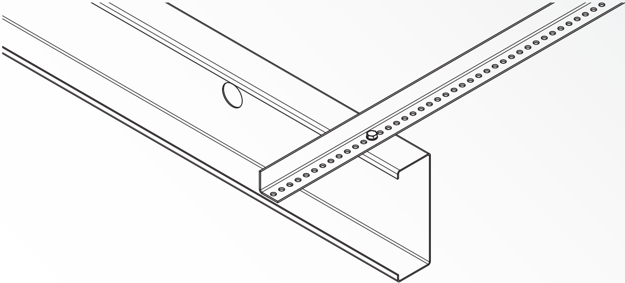
CD-Profil 60/27, z. B. 5120 als Tragprofil für Beplankung Befestigung durch Schnellmontage-Clip 6092
