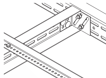
Auswechslung mit Montagewandwinkel 6183 und Montageset 6203
