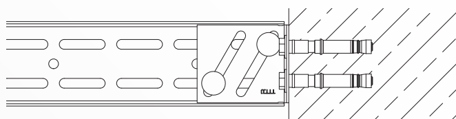
Wandanschluss UA-Profil mit Montagewinkel*
