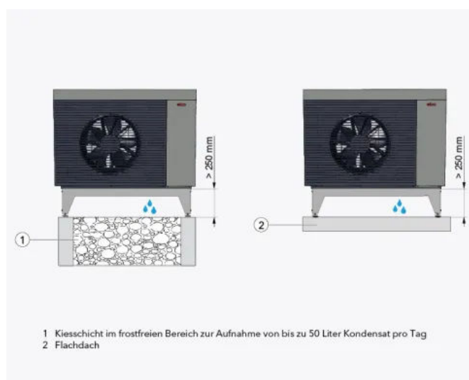
Kondensat frei austropfend, Kiesschicht oder direkt auf das Flachdach
